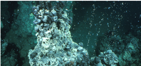
Methan-Karbonat-Turm aus dem Schwarzen Meer mit Methangasblasen
